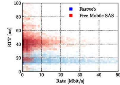
(d) RTT vs throughput: Fastweb and Free
